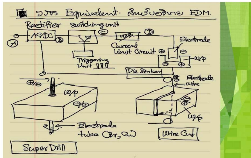
เครื่องสปาร์ค หรือ Electrical Discharge Die Sinking Machine (EDM) แบบ Z-NC และ CNC
